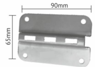
SINGLE SHELF MINI CHANNEL DC-06
