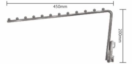
BALENO SOLID HANGER STAND DC-45
